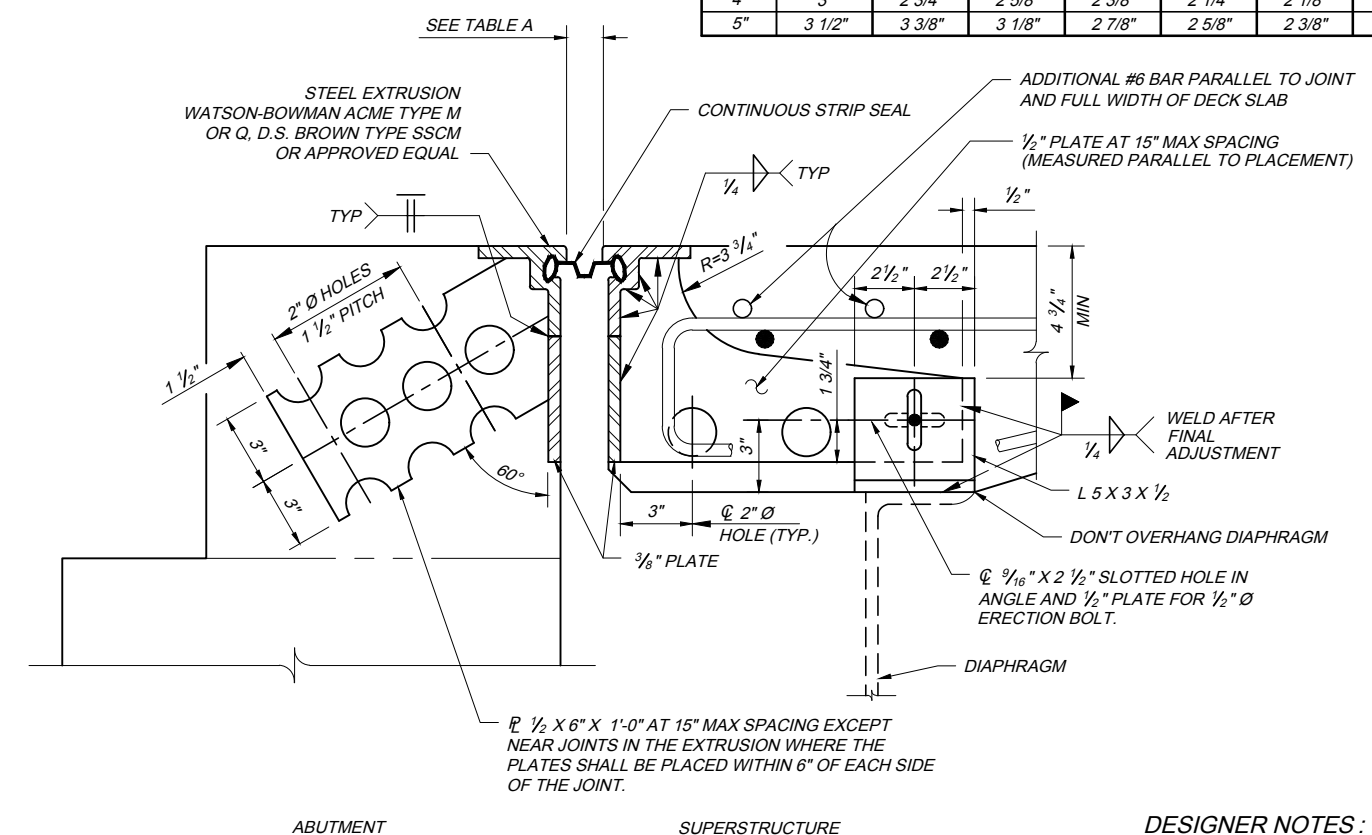
SECTION A-A (STRIP SEAL)
